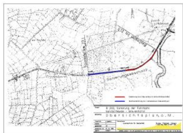
Bild 1: Lageplan
