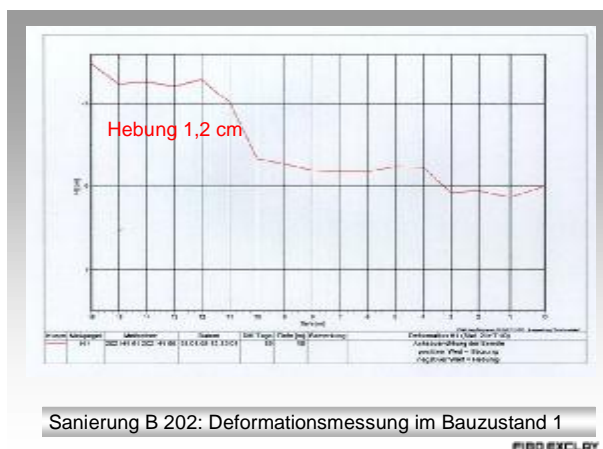
Bild 15: Deformationsmessung Bauzustand 1
