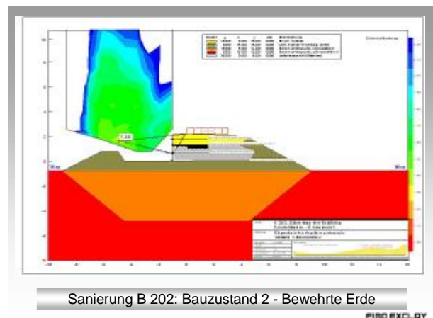
Bild 16: Bewehrte Erde Bauzustand 2
