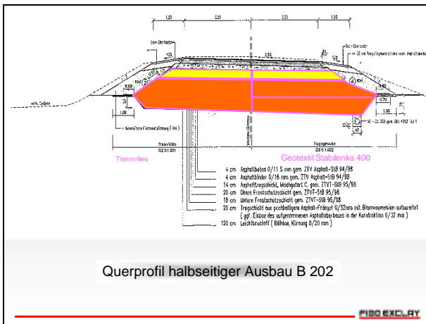
Bild 10: Querprofil
